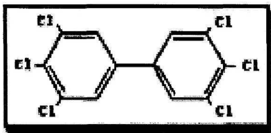
3,3',4,4',5,5'-Hexachlorobiphenyl
