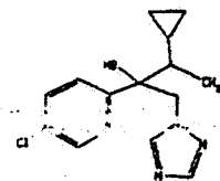
Cyproconazole
