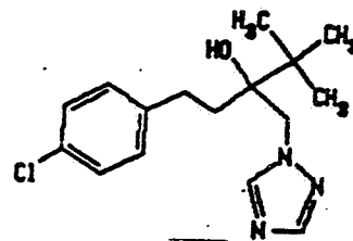
Tebuconazole
