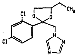
Baycor
