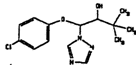
Baytan
