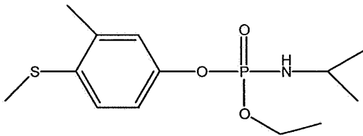
Fenamiphos
