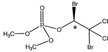
Naled
