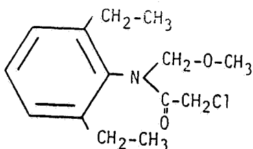
2-Chloro-2',6'-diethyl-N-(methoxymethyl)acetanilide
