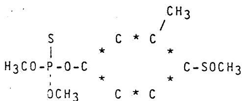
Fenthion
