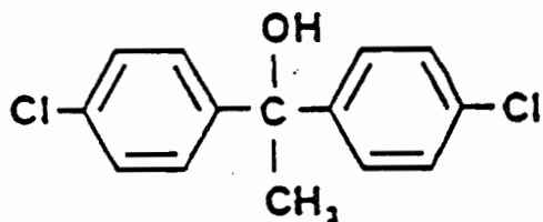
1,1-bis(4-Chlorophenyl)ethanol
