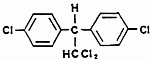
1,1-bis(4-Chlorophenyl)- 2,2-dichloroethane
