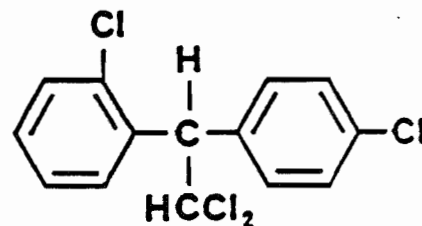
1-(2-Chlorophenyl)-1-(4'-chloro- phenyl)-2,2-dichloroethane
