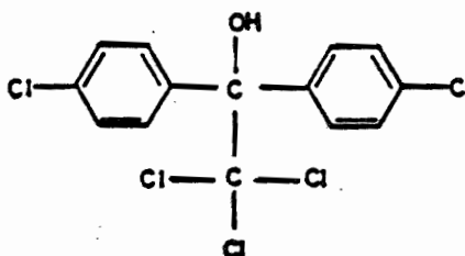
1,1-Bis(p-chlorophenyl)-2, 2,2-trichloroethanol
