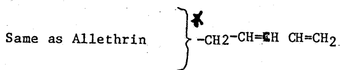
Pyrethrin
