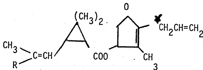
Allethrin
