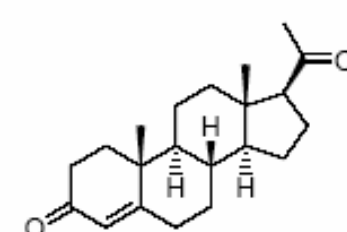
Progesterone
