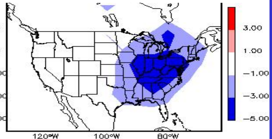
\Delta 2050 \text{ emissions \& } 2050 \text{ climate})
