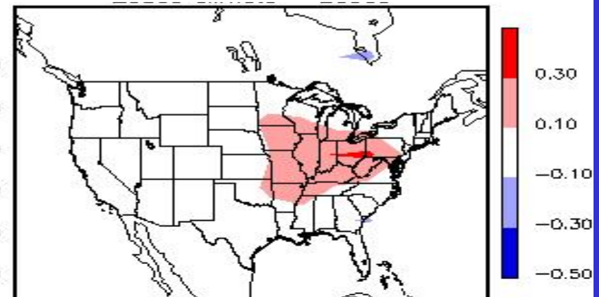
\Delta 2050 \text{ emissions \& } 2050 \text{ climate})
