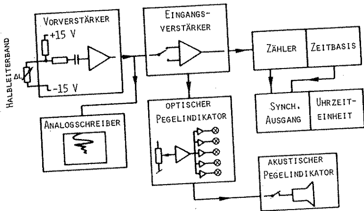
Abb. 2. Die Registrierapparatur
