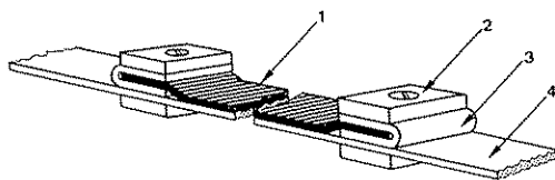
Abb. 1. Dehnungsmessband zur Erfassung der Atembewegungen. 1 = Halbleiterband (Scotch 13 E P R); 2 = Druckplatte; 3 = Kontaktgitter; 4 = Elastisches Trägerband
